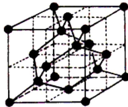
図1 ダイヤモンド構造の単位格子
