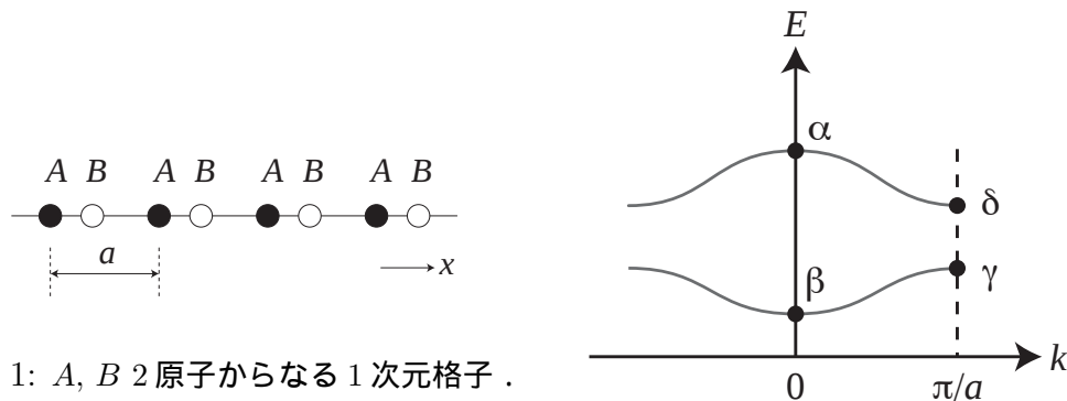
図 2: AB 1 次元格子のエネルギーバンド. ただし, k は波数を表す.
