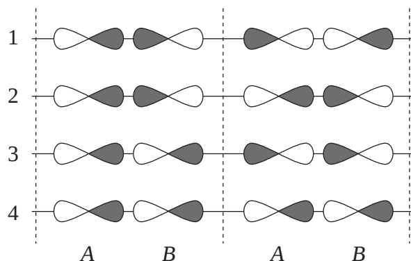
図 3: 1 次元格子における A , B 原子の p_x 軌道の模式図.
