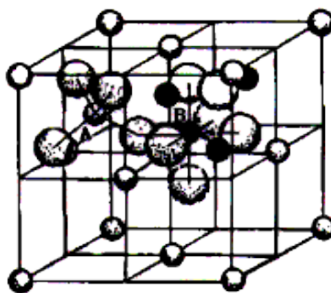
図1 スピネル型構造の単位格子。図中、小さい白丸、黒丸はそれぞれAサイト、Bサイトの金属イオンを、大きい丸はCサイトの陰イオンを表している。
